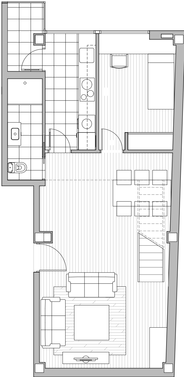
Planta 1
