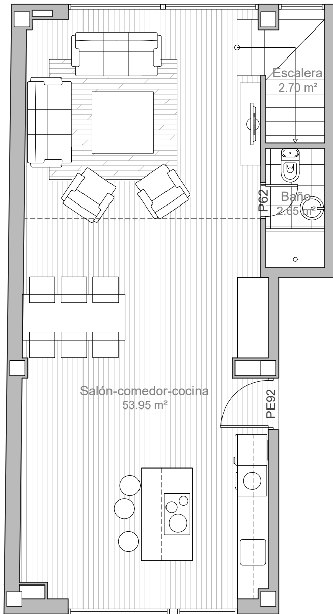
Planta 2
