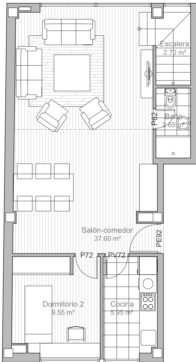
Planta 2
