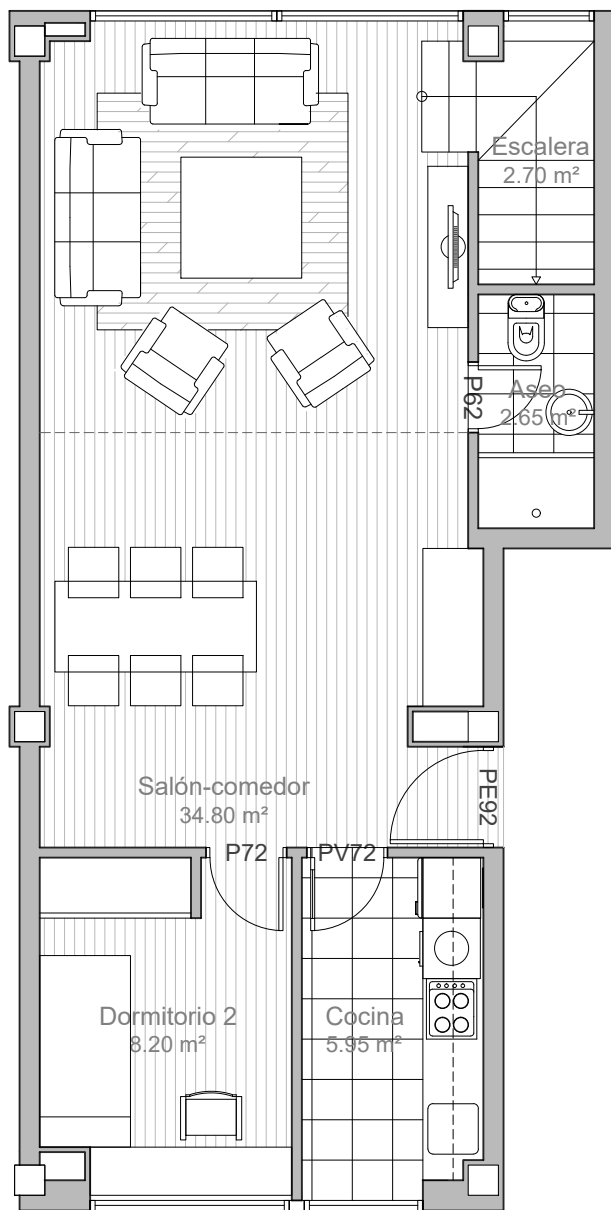
Planta 2
