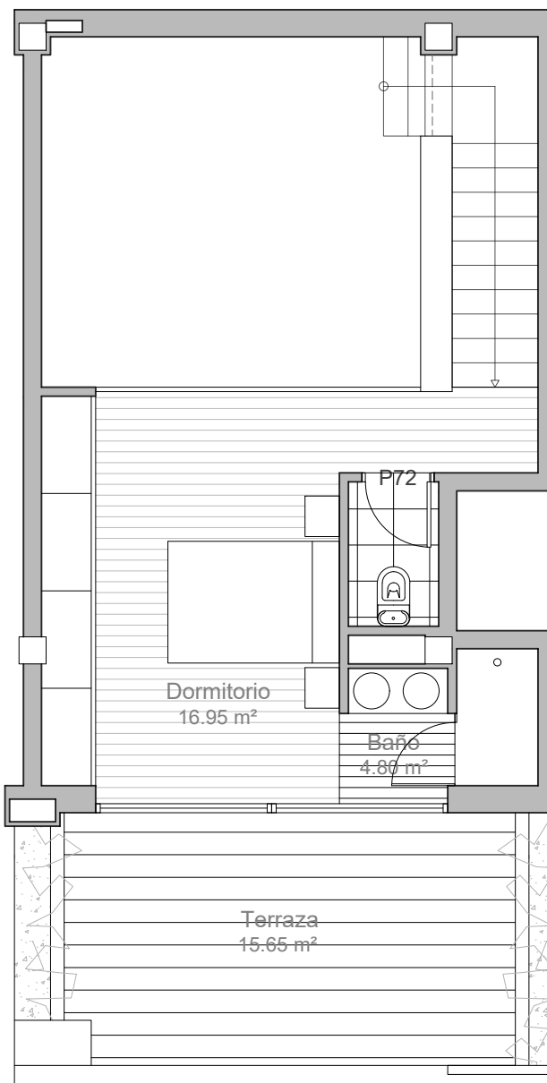
Planta ático
