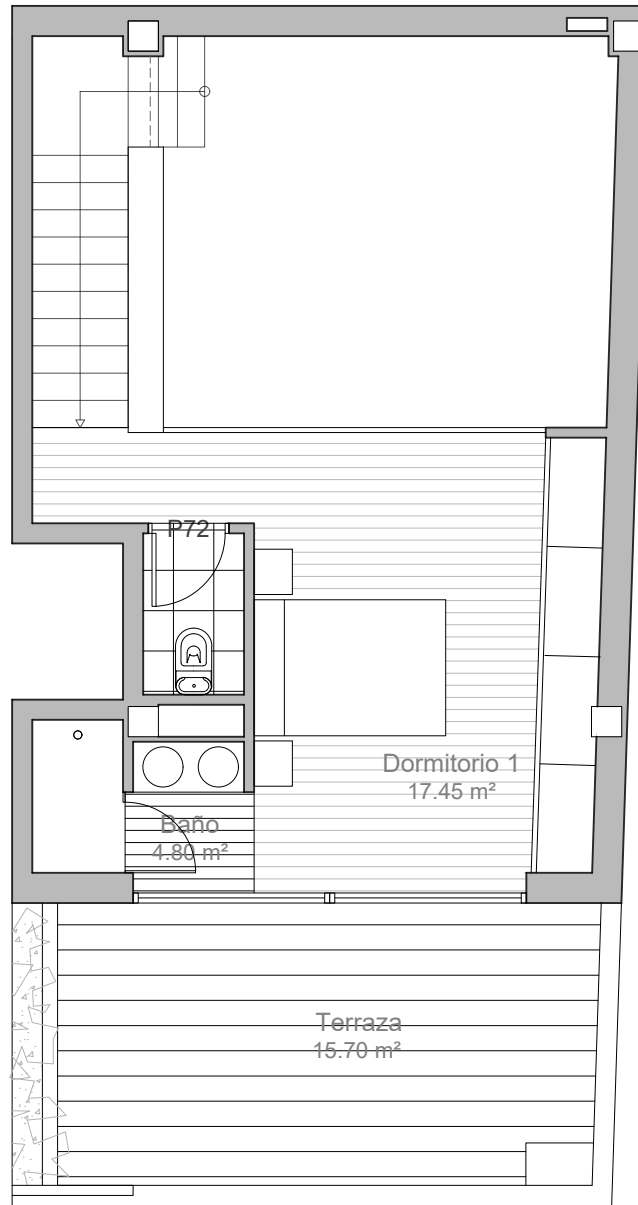
Planta ático
