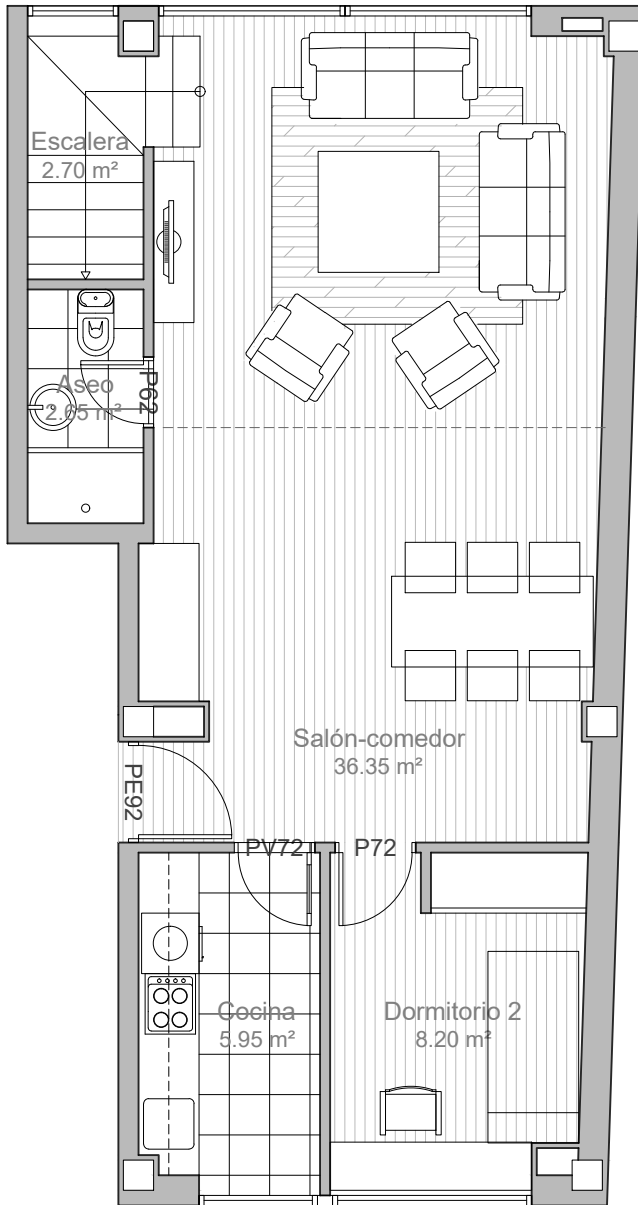
Planta 2
